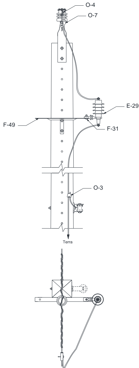
Figura 108 – Instalação de equipamento – Para-raios – Estrutura monofásica – 2º nível
