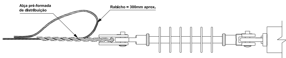
Opção de ancoragem simples sem gancho-olhal
